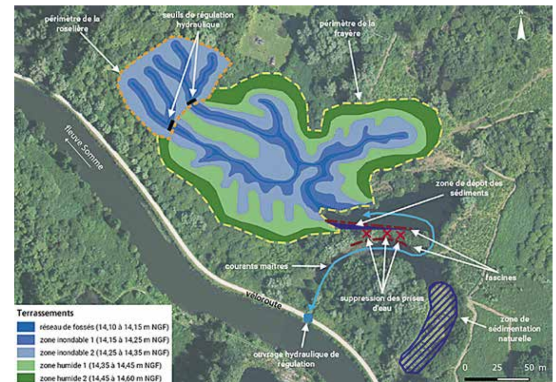
Figure 1 - Plan des aménagements et terrassements
